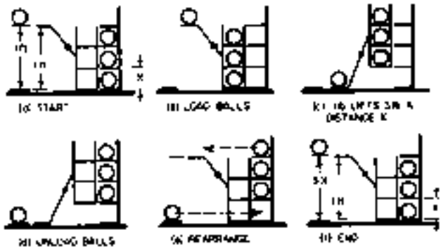
(དཔེ་རིས་ ༡) སྤྱིར་སློབ་འཕུལ་འཁོར། (A reversible machine)
