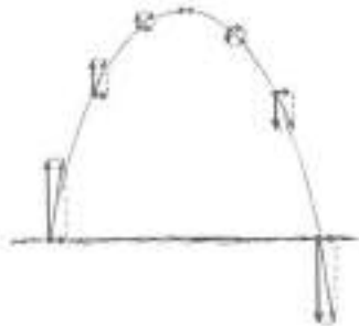
(དཔེ་རིས་ ༡༩ ཟུར་ཁྲུག་གཟར་པོར་འཕེན་པའི་འཕེན་གཟུགས་ཀྱི་ལམ་)
