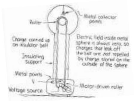
( དཔེ་རིས་ ༩༠ : མཚུངས་ཀྱི་རྗེས་སློག་འདོན་འཕུལ་འཁོར་གྱི་དཔེ་གཟུགས་སྐབས་བདེ་ཞིག )
