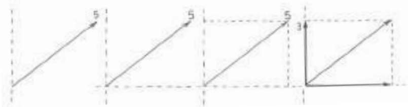
(དཔེ་རིས་ 6 སྤྱིགས་ལྗོངས་ཤིག་གི་རང་གི་ཆ་གཅིག་ལས་འབྲེད་དང་གཞུང་གི་བྱུང་སྟངས་)
